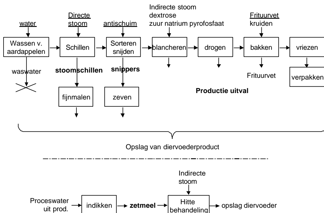
Figuur 1 Processchema aardappelproducten.
